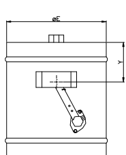
SEZIONE (pala chiusa)
